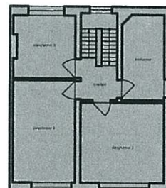
nivo +2 - app.2 bruto 75,6m 2 schaal: 1cm = 75cm
