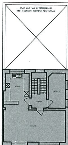
nivo +1 - app.2 bruto 75,6m 2 schaal: 1cm = 75cm
