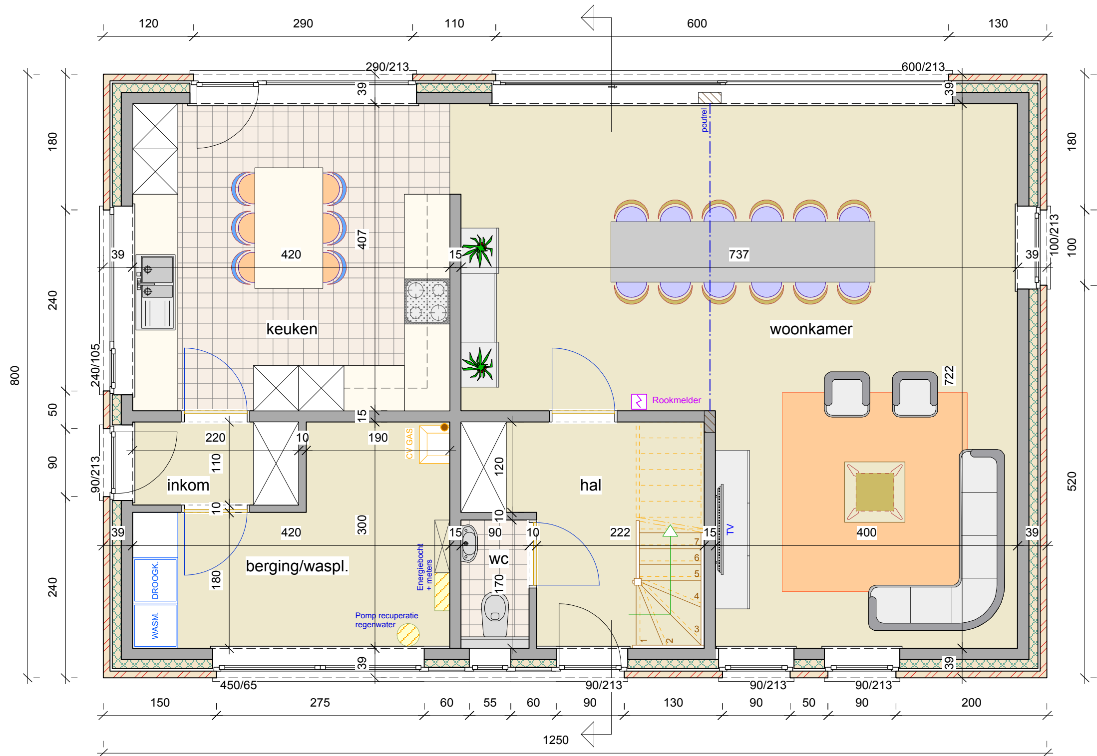
Plan GELIJKVLOERS
