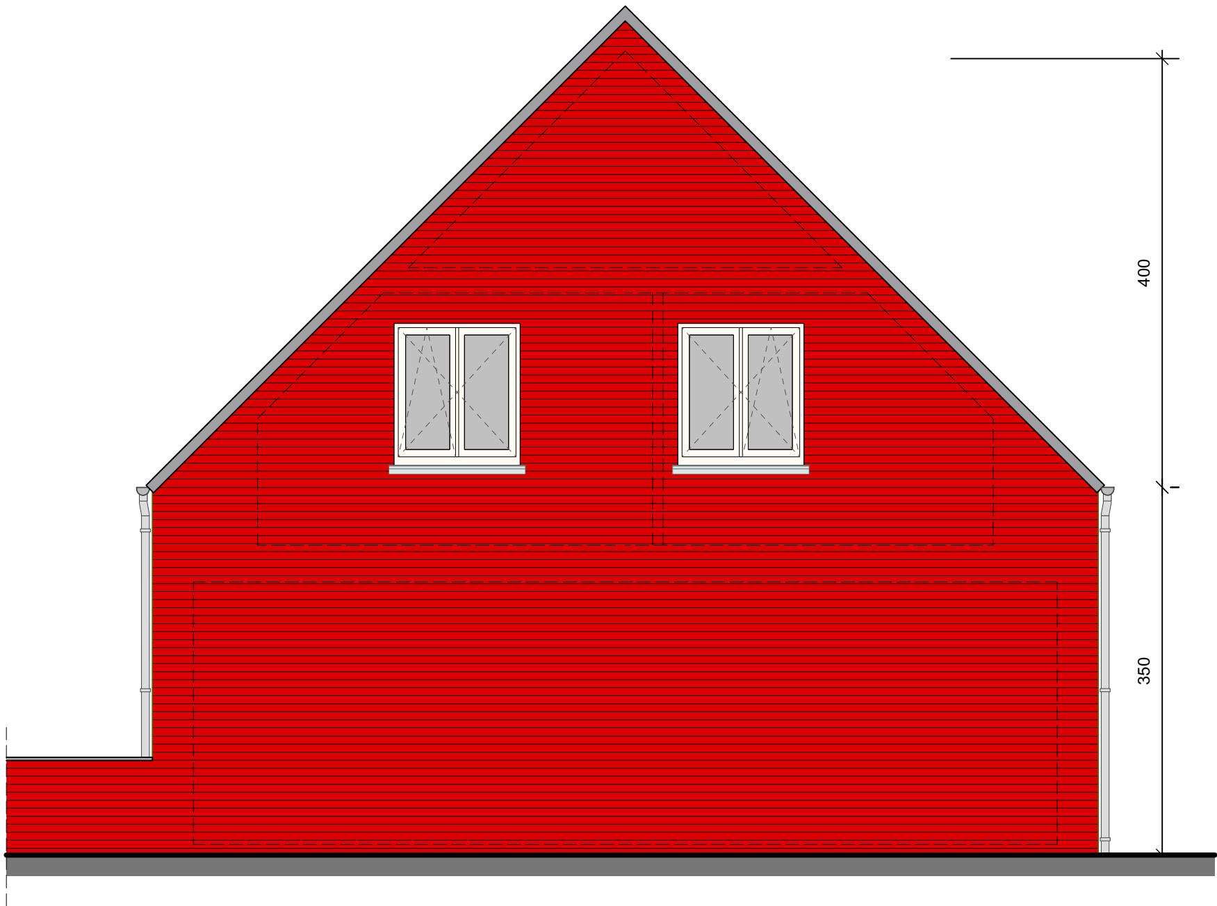
Zijgevel rechts
